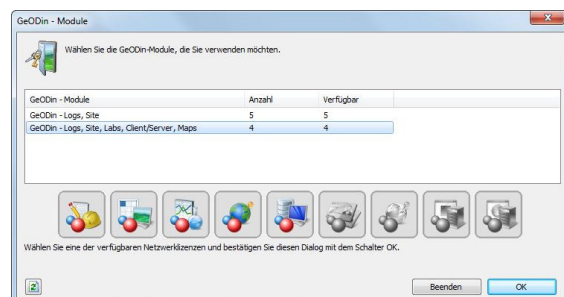
Schritt 6: Lizenzauswahl
